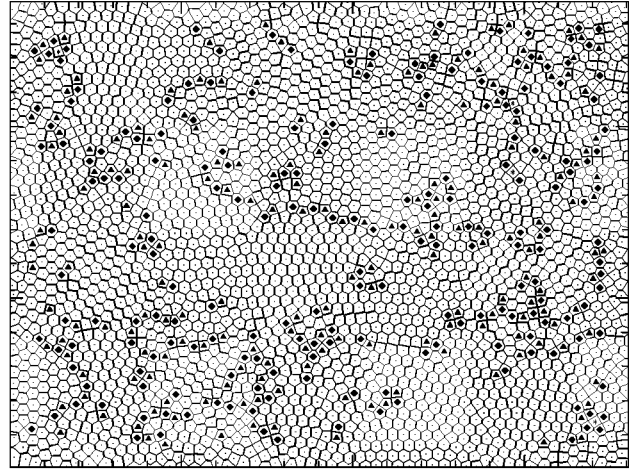
(d) disclination concentration = 0.35
