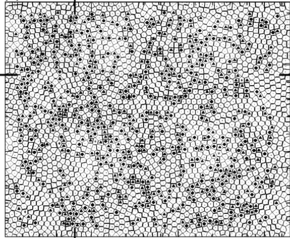
(d) disclination concentration = 0.35
